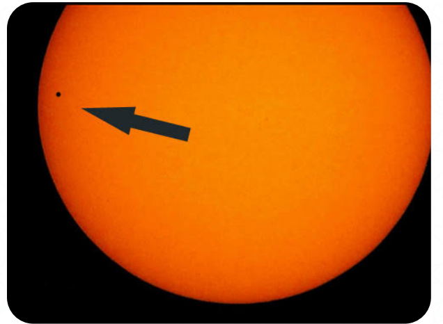
11 Kasım 2019 tarihindeki transit geçişi sırasında Utarid
