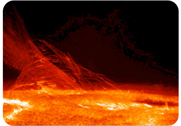
Güneş yüzeyindeki spiküller. Bu spiküller, Güneş yüzeyinin üzerinde koyu renkli “tüyler” gibi görünürler.
