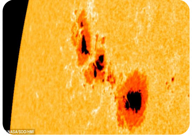
Güneş lekelerinin daha yakından görünüşü
