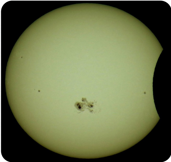
Ay Tutulması başlangıcında gözlemlenmiş Güneş lekeleri
